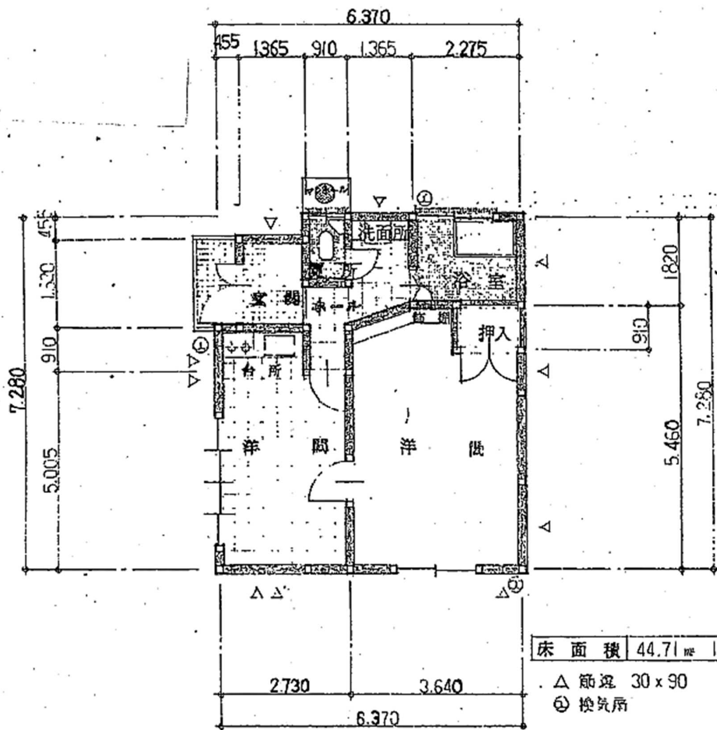
平 面 図 1:100
