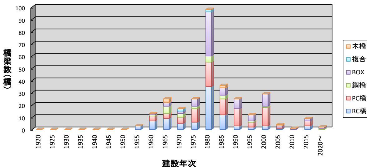
図-1 架橋年別の橋梁数分布
