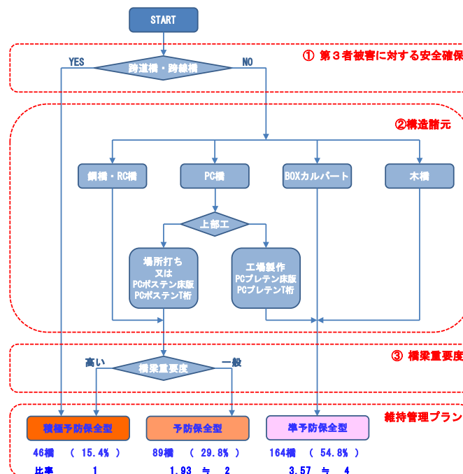
図-4 維持管理プランの設定フロー
