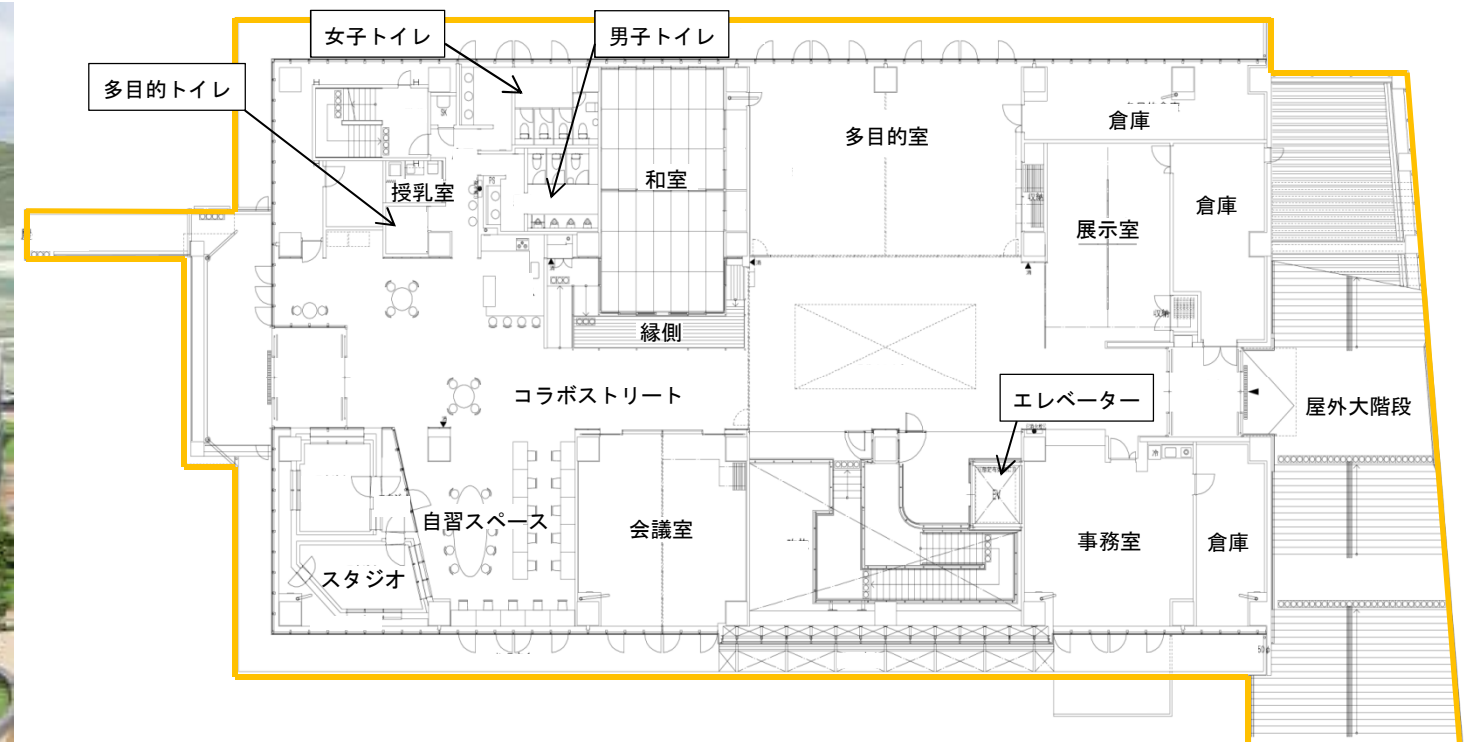
2 階平面図
