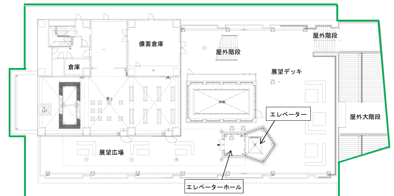
3 階平面図
