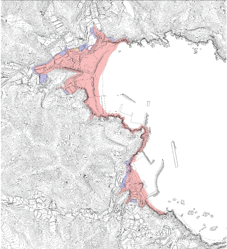
災害危険区域図（12：野々前・白浜地区）
