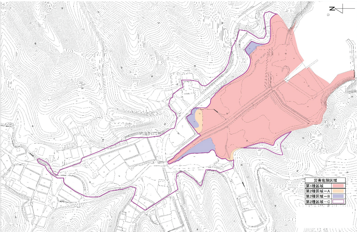
災害危険区域図（15:合足地区）
