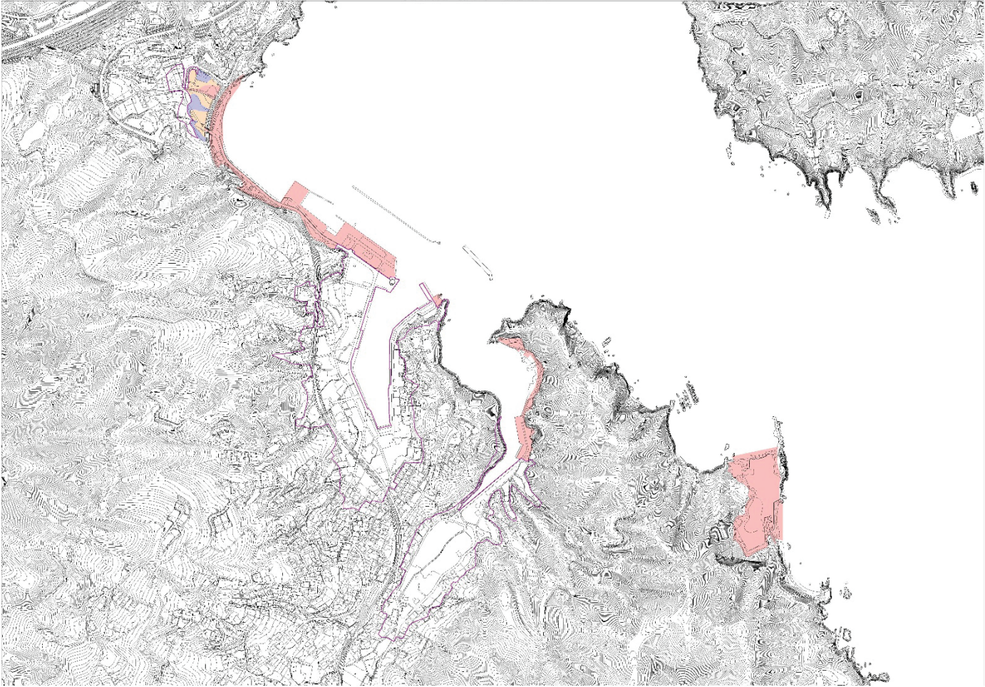
災害危険区域図（22:細浦地区）
