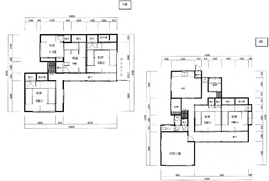
間取り
