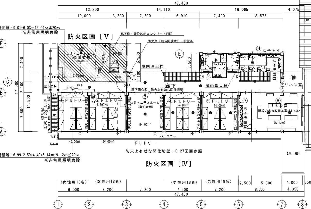
――は歩行距離を示す(2階20m以内は居室非常用照明免除) 2 階 平 面 図 S=1:250 ●は非常用照明を示す 【西棟2階 658.13m 2 】 ※Fは随時閉鎖式防火戸
