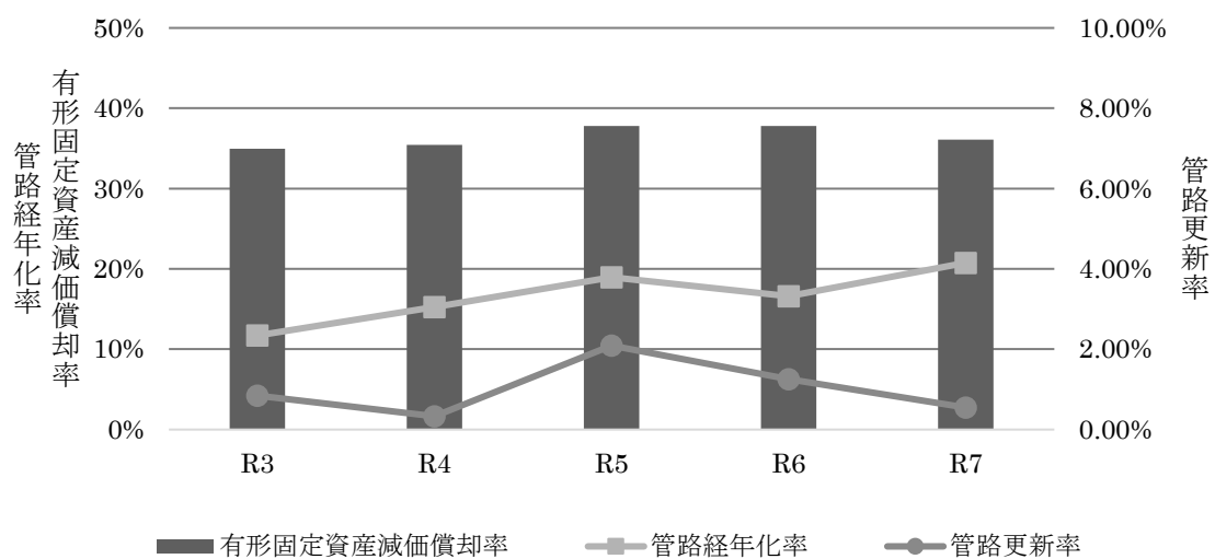
有形固定資産減価償却率・管路経年化率・管路更新率の推移
